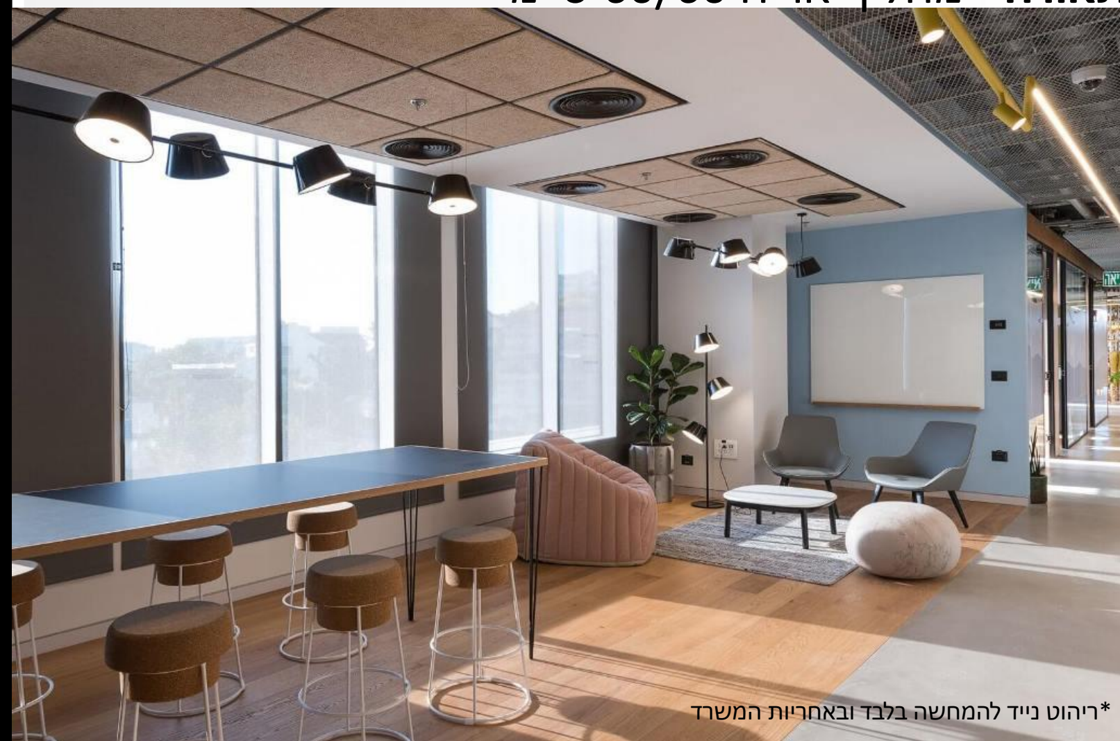
תקרה - לוחות צמר עץ בתלייה מונחת פריקה במידות 60*60 ס"מ פרופיל שחור תאורה - מחליף אריח 60/60 ס"מ
